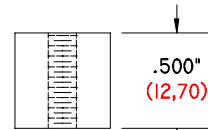
GI-500-500/8-32 DS .500" (12,70) LONG .500" (12,70) Ø O. D. 8-32 THREAD DELRIN SPACER
