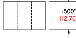
GI-500-750/257 DS .500" (12,70) LONG .750" (19,05) Ø O. D. .257" (6,53) Ø I. D. DELRIN SPACER
