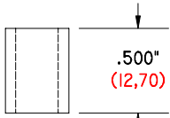
GI-500-375/257 DS .500" (12,70) LONG .375" (9,53) Ø O. D. .257" (6,53) Ø I. D. DELRIN SPACER
