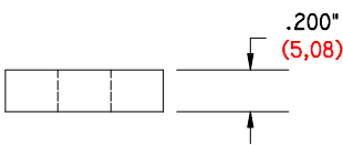
GI-200-750/257 DS .200" (5,08) LONG .750" (19,05) Ø O. D. .257" (6,53) Ø I. D. DELRIN SPACER
