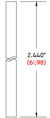
GI-2440-187 FL 2.440" (61,98) LONG .187" (4,75) Ø O. D. DELTRIN POST
