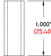
GI-1000-375/257 DS 1.000" (25,40) LONG .375" (9,53) Ø O. D. .257" (6,53) Ø I. D. DELTRIN SPACER
