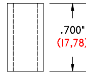
GI-700-375/257 DS .700" (17,78) LONG .375" (9,53) Ø O. D. .257" (6,53) Ø I. D. DELTRIN SPACER
