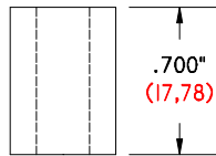
GI-700-500/257 DS .700" (17,78) LONG .500" (12,70) Ø O. D. .257" (6,53) Ø I. D. DELTRIN SPACER
