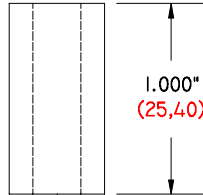
GI-1000-500/257 DS 1.000" (25,40) LONG .500" (12,70) Ø O. D. .257" (6,53) Ø I. D. DELTRIN SPACER
